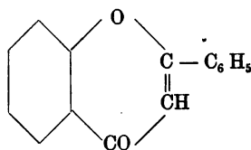
Flavon.
